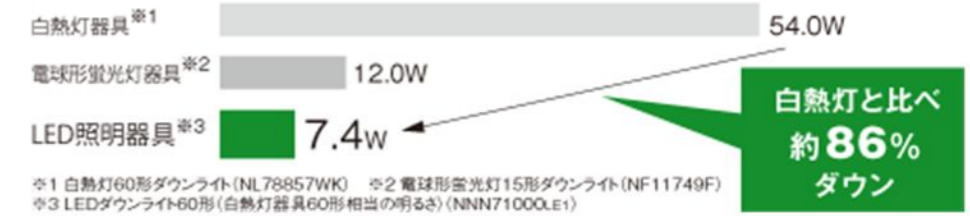
■同じ明るさの器具1台あたりの光源別消費電力量比較
